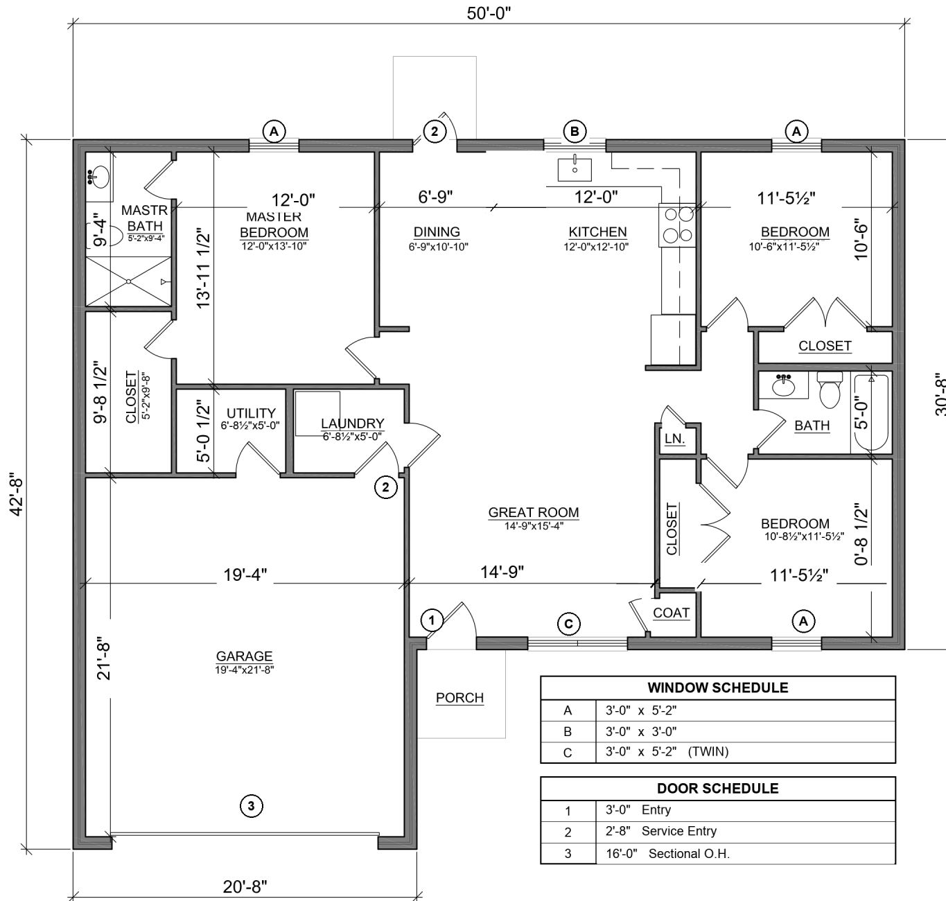
A FLOOR PLAN A1.1 SCALE: 1/8" = 1'-0"
